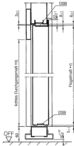
Variante Schlupftür mit 60mm Schwelle *1)
