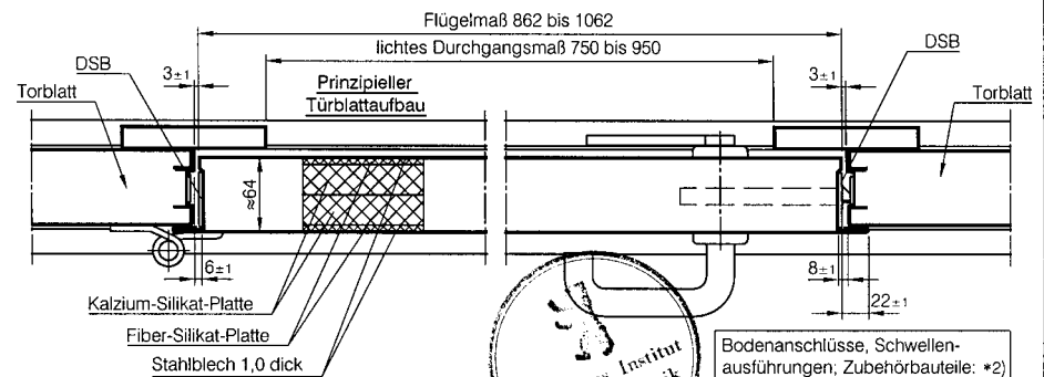
Variante Schlupftür mit 20mm Schwelle *1)
