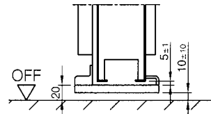
Variante Schlupftür mit 20mm Schwelle *1)
